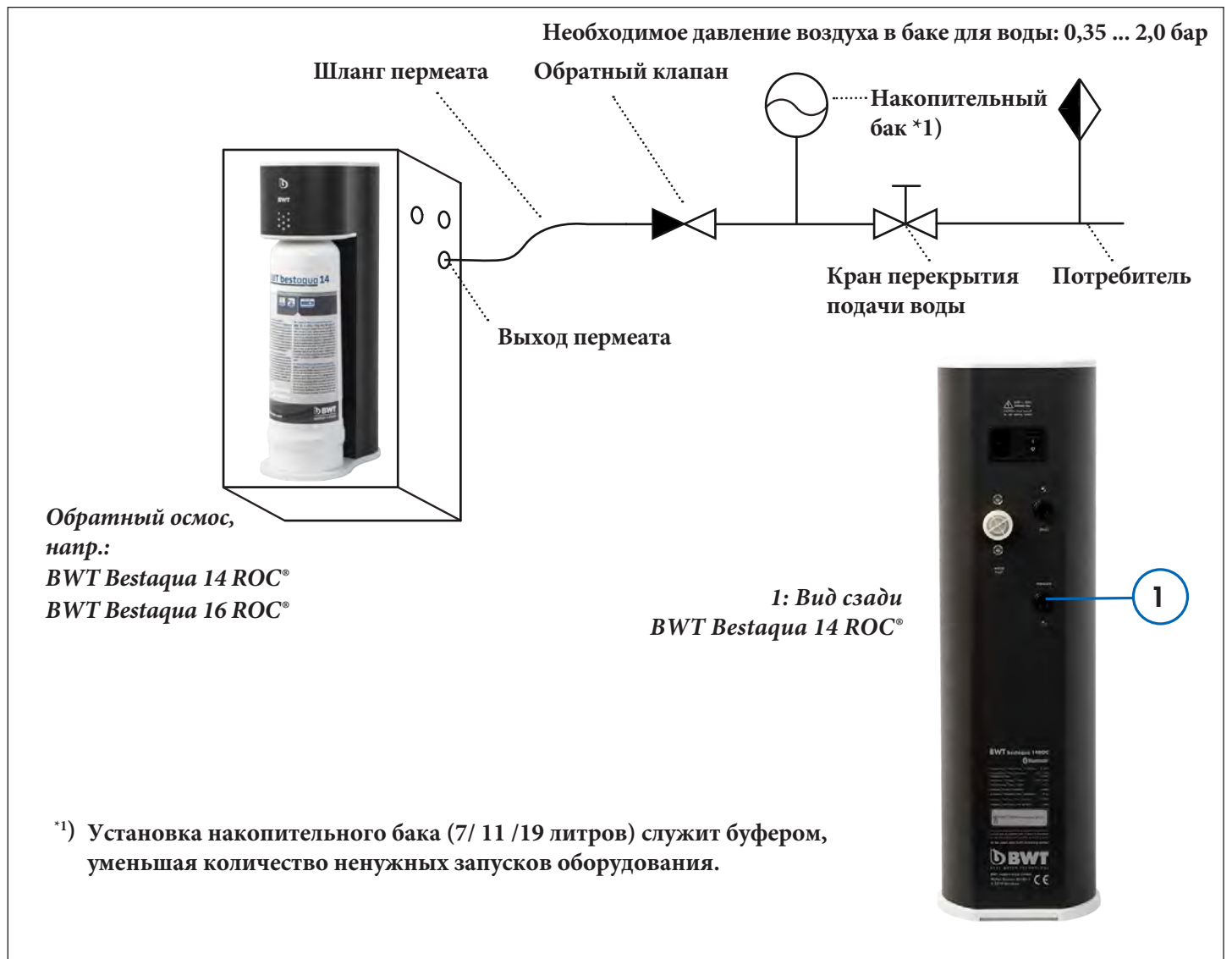
Рис. 4: Схема установки комплектов накопительных баков BWT к потребителю
